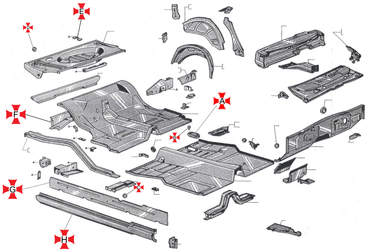
ASSOALHO E PAINEL DIANTEIRO
