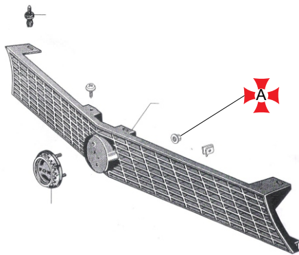
GRADE DO RADIADOR
