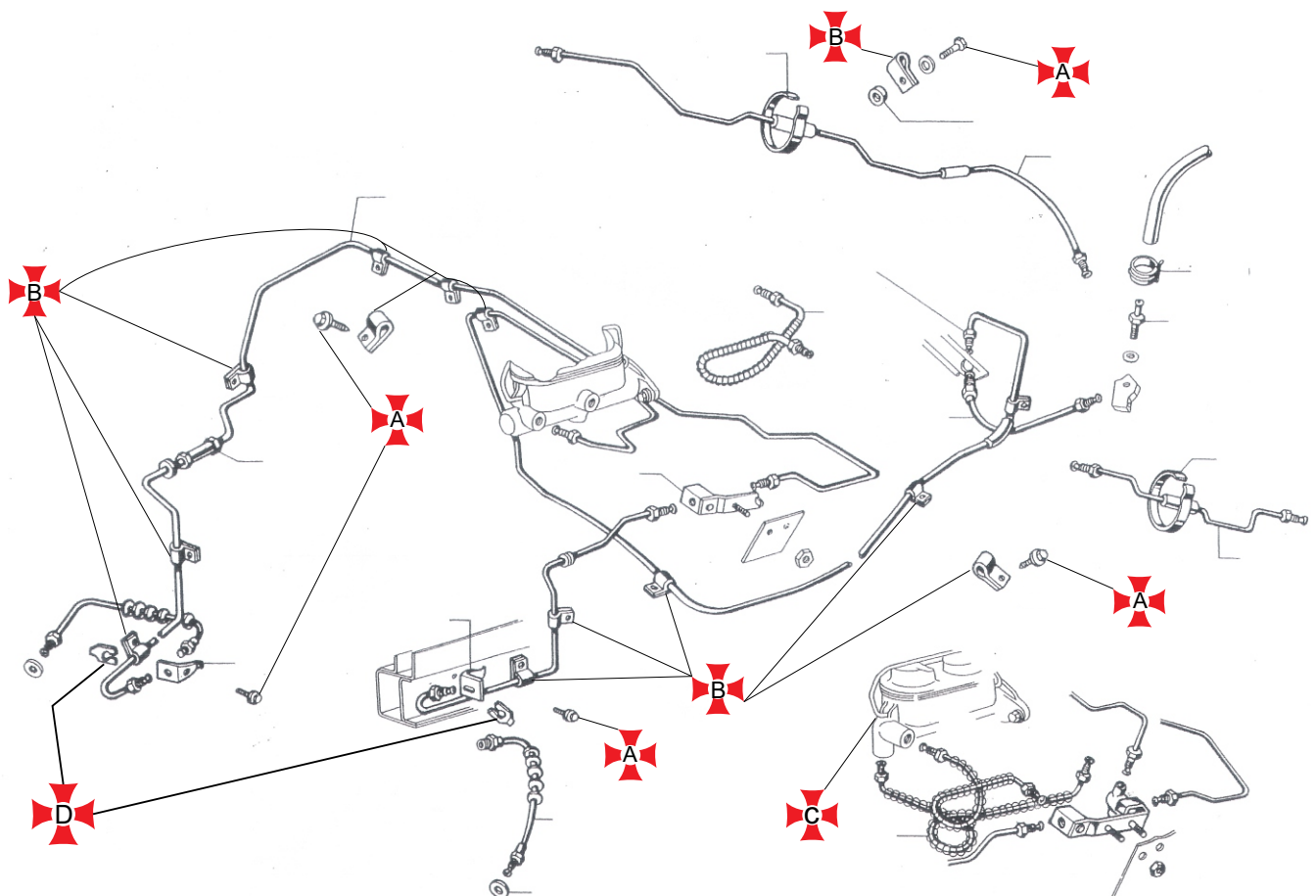
TUBULAÇÕES DO SISTEMA DE FREIOS
