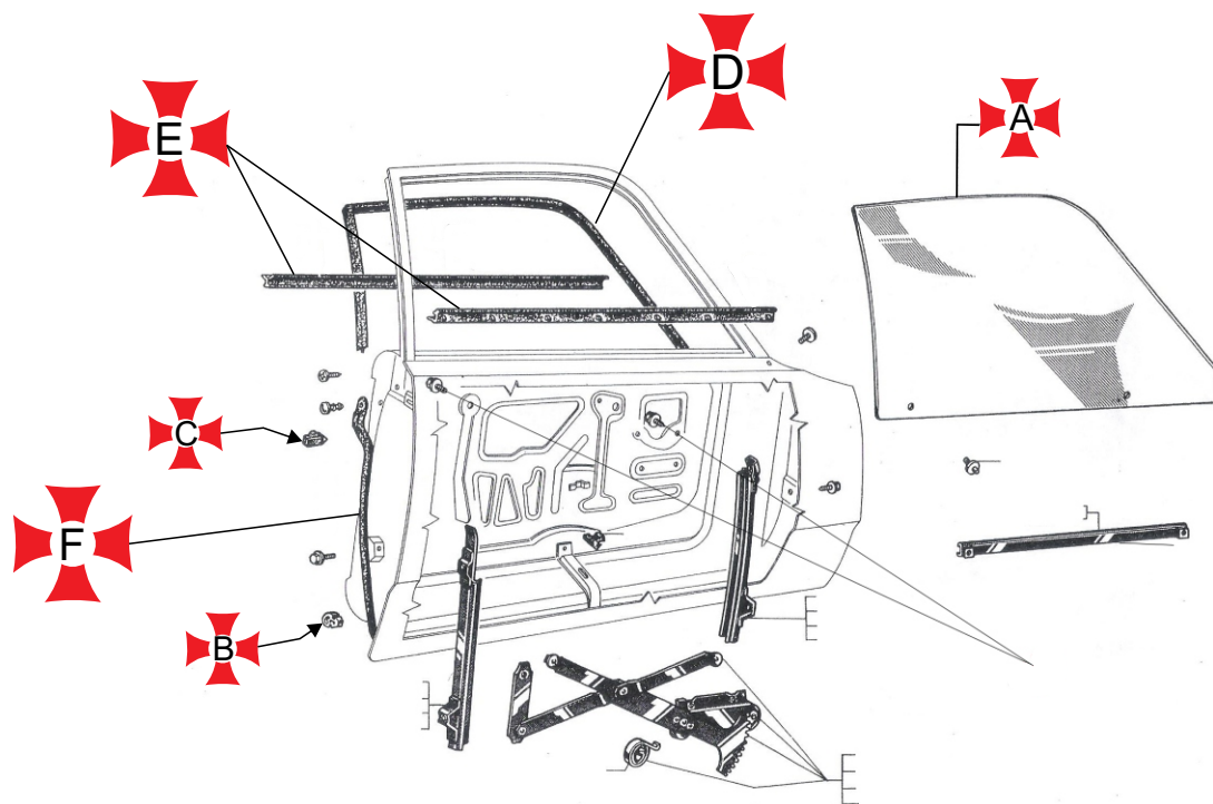
JANELA E MECANISMO DA PORTA DIANTEIRA
