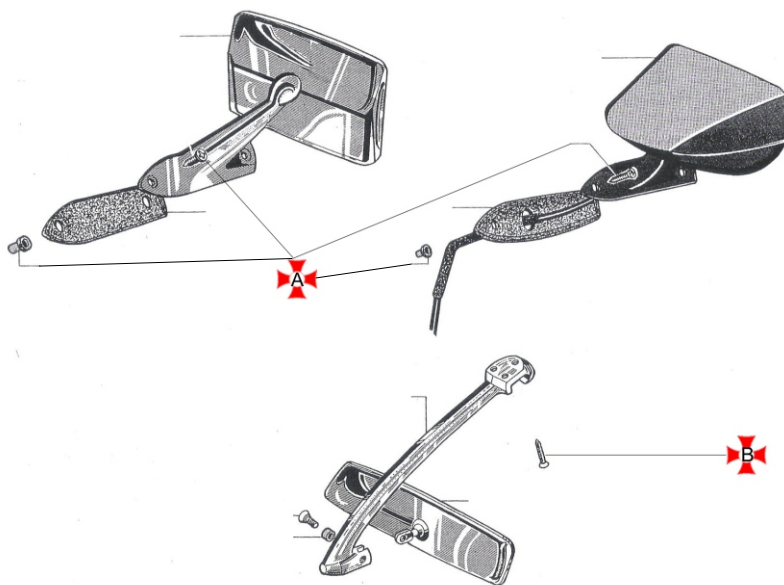
ESPELHOS RETROVISORES—EXTERNO E INTERNO
